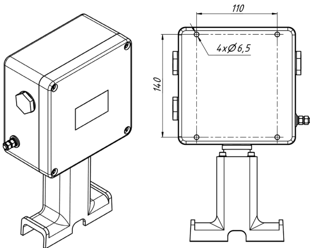
Установочные размеры
