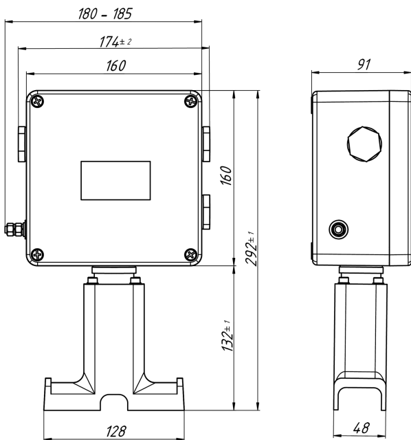
Габаритные размеры
